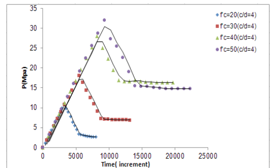
شکل ۲۸: فشارهای وارد بر آرماتور برای c/d=4 و فشار اولیه P=2.5 MPa Fig.28. Pressures on bars at c/d=4 and P=2.5 MPa
