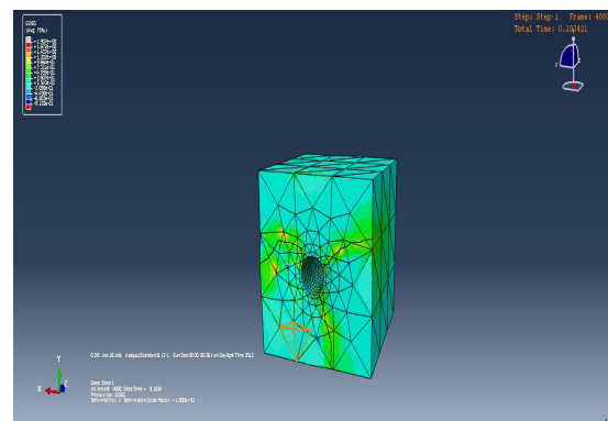
شکل ۱۳: مقایسه نمونه ترک خورده آزمایشگاهی با روند رشد ترک در مدل طراحی شده (آرماتور در وسط)
