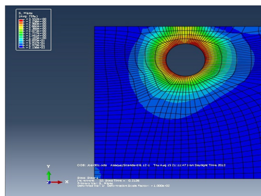
شکل ۸: توزیع تنش شعاعی اطراف آرماتور (مدل عددی)
