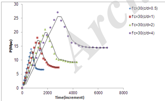
شکل ۳۰: فشارهای وارد بر آرماتور برای f_c=30 در فشار ۵ MPa Fig.30. Pressures on bars at f_c=30 and P=5 MPa
